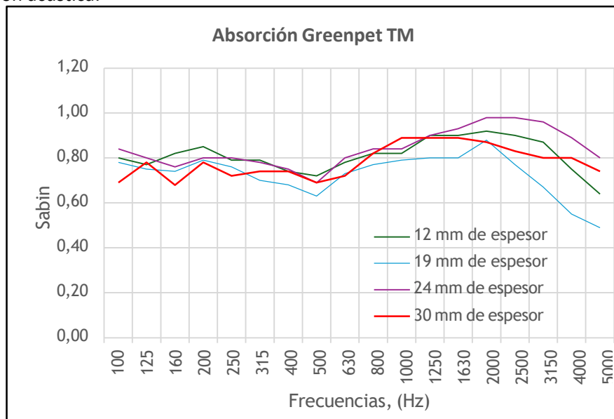
Segun Norma ASTM ISO 354. Camara de aire de 400 mm.
